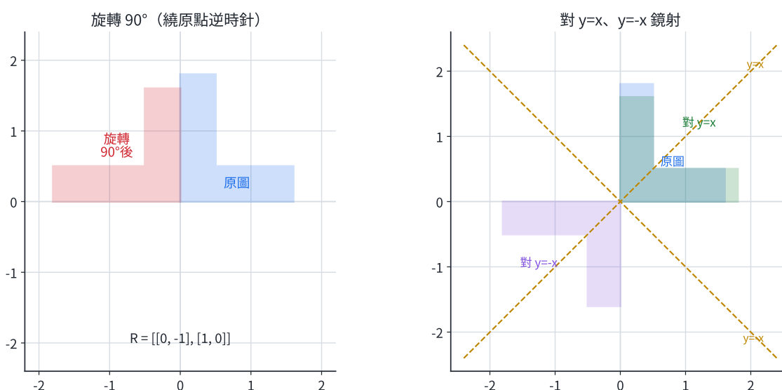
圖 2-4：旋轉（繞原點逆時針轉 \theta ，左）與兩條對角線鏡射（對 y = x 、對 y = -x ，右）。旋轉的 \det = 1 、鏡射的 \det = -1 （負號代表把定向翻面），兩者都不改變面積。
